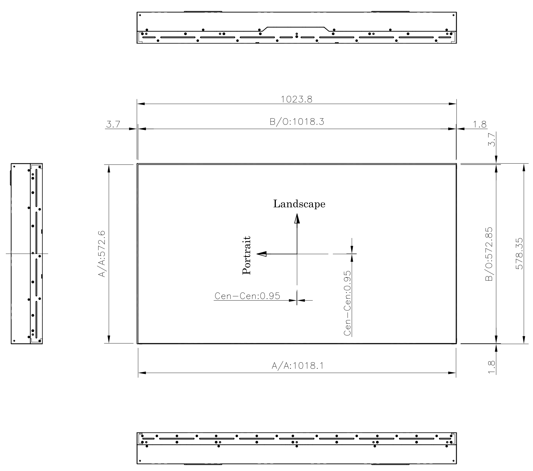
① D46KFA Display
