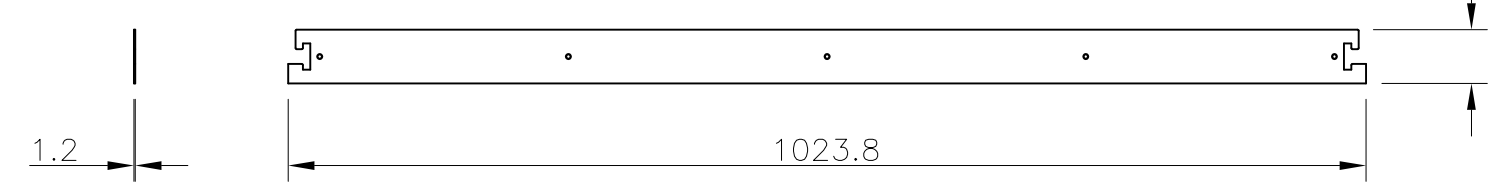
②-2) Muiti Brkt Ver < Multi Display > (Brkt-2Ea)
