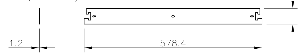
②-2) Muiti Brkt Ver < Multi Display > (Brkt-2Ea)
